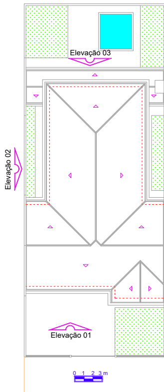
Implantação e Cobertura
