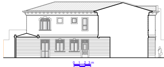
Elevação 02
