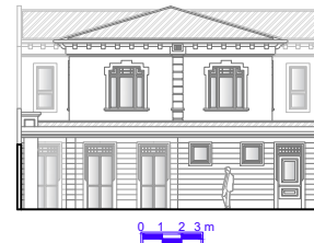
Elevação 03
