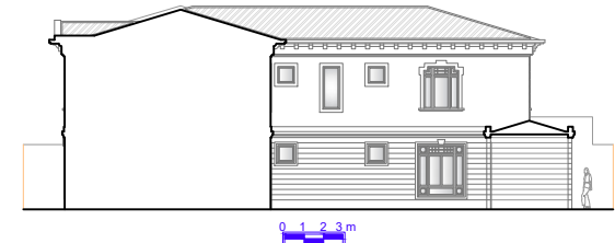
Elevação 04
